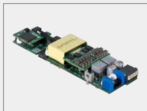
单插槽双输出 (最大240W输出)
