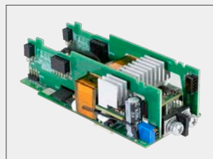
三插槽单输出 (最大1200W输出)
